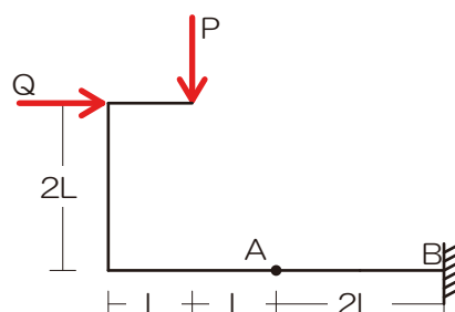
固定支点
